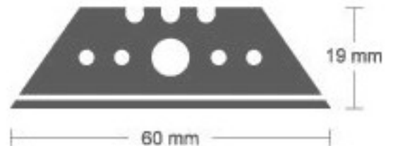
Lame trapèze en acier supérieur 19 x 60 mm
